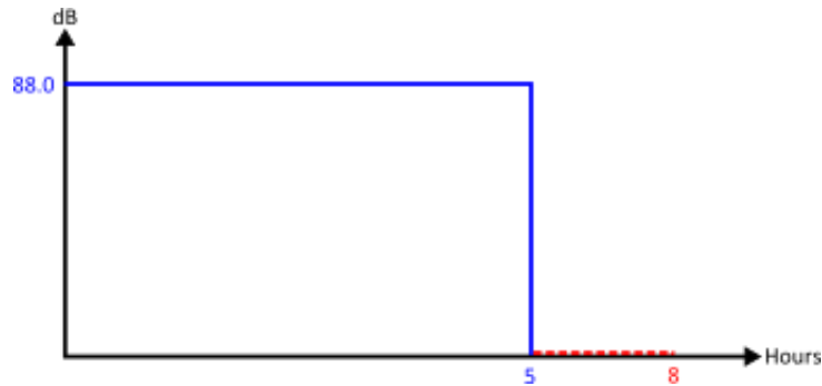
La figura 9 muestra la medición de 5 horas (línea azul); no hay exposición adicional al ruido durante el resto del periodo de 8 horas (línea roja)
