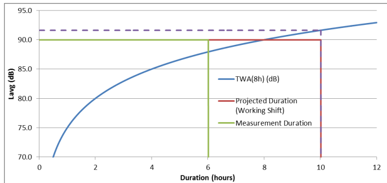
La figura 5 muestra una medición de 6 horas (línea verde); esto se proyecta hacia delante, hasta el final de las 10 horas de jornada laboral (línea roja); el lugar en el que el valor proyectado cruza la TWA(8h) original (línea azul) es donde se encuentra la TWA(8h) real, indicada por una línea discontinua.
