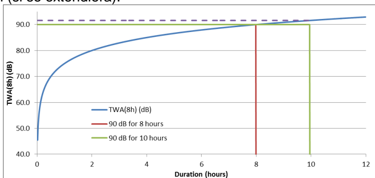
La Figura 3 muestra que el valor de la TWA(8h) es superior a 90 dB cuando la jornada laboral es de 10 horas (el valor de la TWA(8h) corresponde al punto donde la línea azul cruza la línea verde, si se extendiera esta línea verde).
