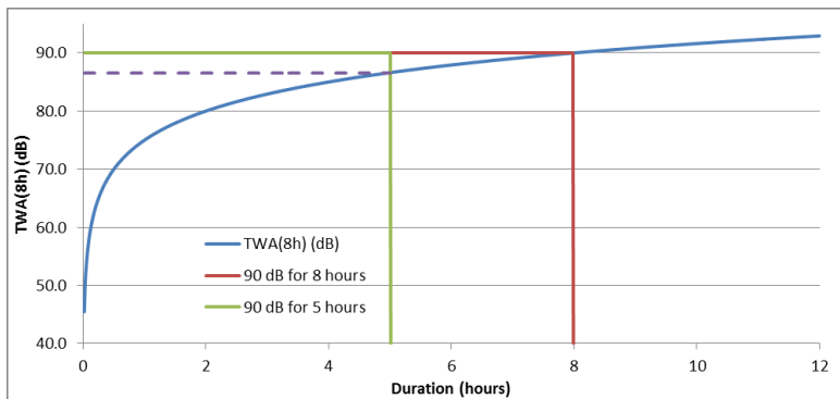
La Figura 2 muestra que el valor de la TWA(8h) es inferior a 90 dB cuando una jornada laboral es de 5 horas (el valor de la TWA(8h) corresponde al punto donde la línea azul cruza la línea verde).
