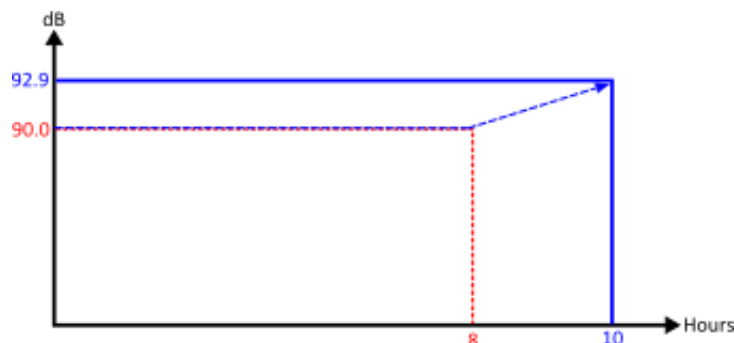
Figura 17 Cuando se calcula la TWA(8h) proyectada, el valor es igual al Lavg mientras el tiempo de medición no supere las 8 horas. Cuando la duración supere las 8 horas, la TWA(8h) empezará a aumentar.
