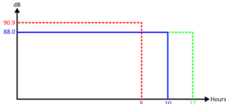
La figura 15 muestra la medición de 10 horas (línea azul); pero también el mismo nivel de ruido continuado durante el resto de la jornada de 12 horas (línea verde). También se muestra la TWA(8h) (línea roja), que tiene la misma energía medida que la representada por la línea verde.
