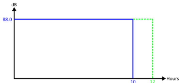
La figura 14 muestra la medición de 10 horas (línea azul); pero también el mismo nivel de ruido continuado durante el resto de la jornada de 12 horas (línea verde)
