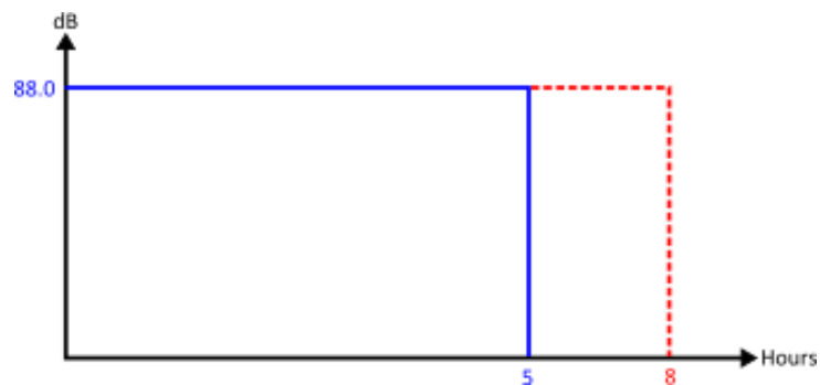
La figura 7 muestra la medición de 5 horas (línea azul); pero también el mismo nivel de ruido continuado durante el resto de la jornada de 8 horas (línea roja)
