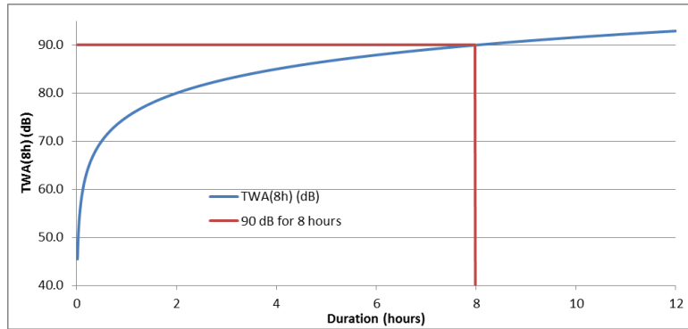
La figura 1 muestra como el valor de la TWA(8h) cambia cuando cambia la jornada laboral.
