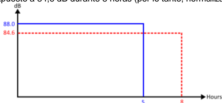
La figura 10 muestra la medición de 5 horas (línea azul); la TWA(8h) está indicada por la línea roja. La energía medida representada por la línea azul es igual a la energía medida representada por la línea roja.
