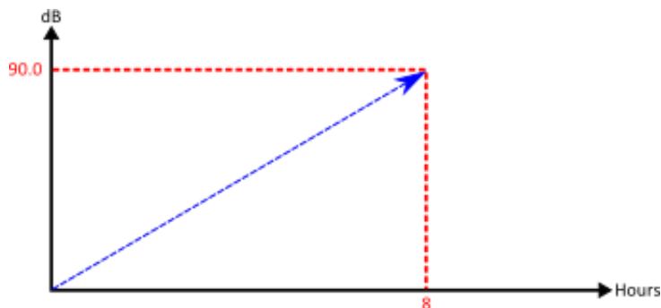
Figura 16 Cuando se calcula la TWA(8h) estándar, el valor aumenta a medida que se incrementa la duración de la medición.
