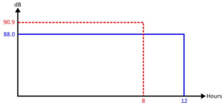
La figura 12 muestra la medición de 12 horas (línea azul); la TWA(8h) está indicada por la línea roja. La energía medida representada por la línea azul es igual a la energía medida representada por la línea roja.
