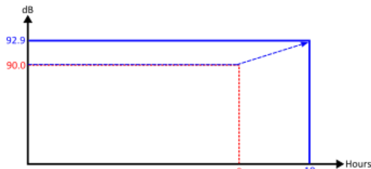
图 17 当计算预期 TWA(8h) 时，当测量时间不大于 8 小时时，该值实际上等于 L_{avg} 。一旦时间超过 8 小时， TWA(8h) 将开始增大。
